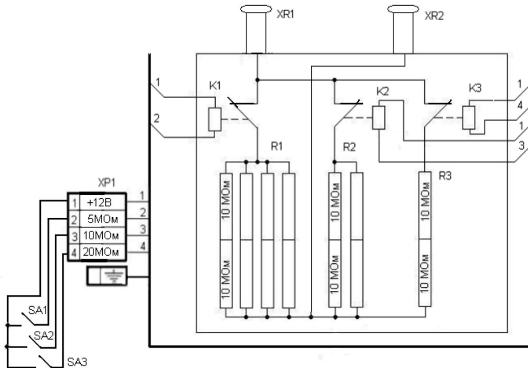
Рис 1. Нагрузка НПВ с 4 номиналами резисторов
