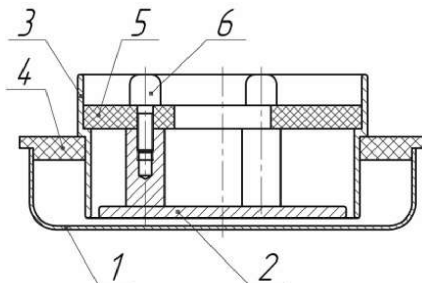
Рисунок 5. Ячейка измерительная:
