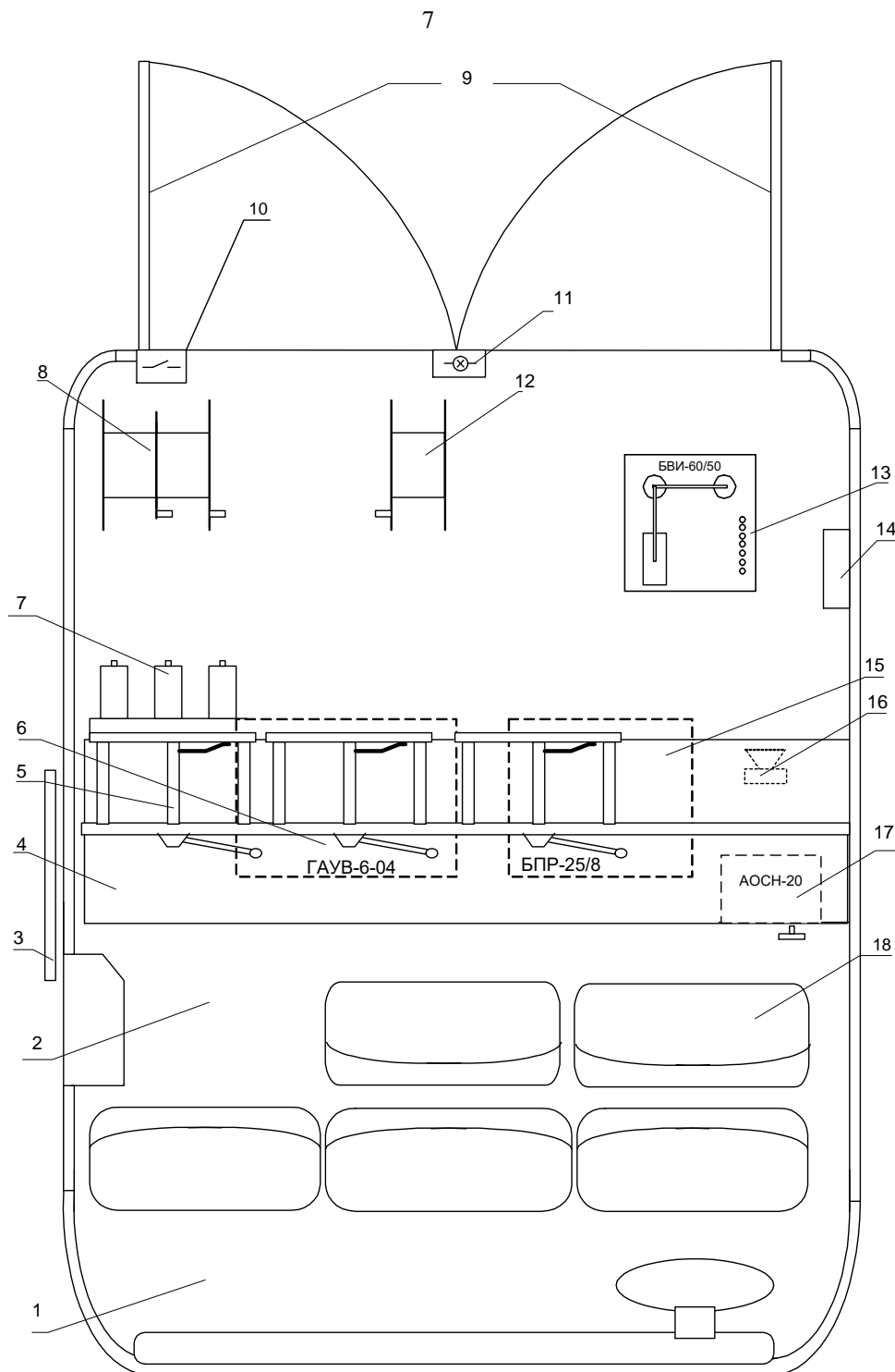
Рис.1. Схема размещения оборудования лаборатории ЭТЛ-10 №77 в фургоне автомобиля
